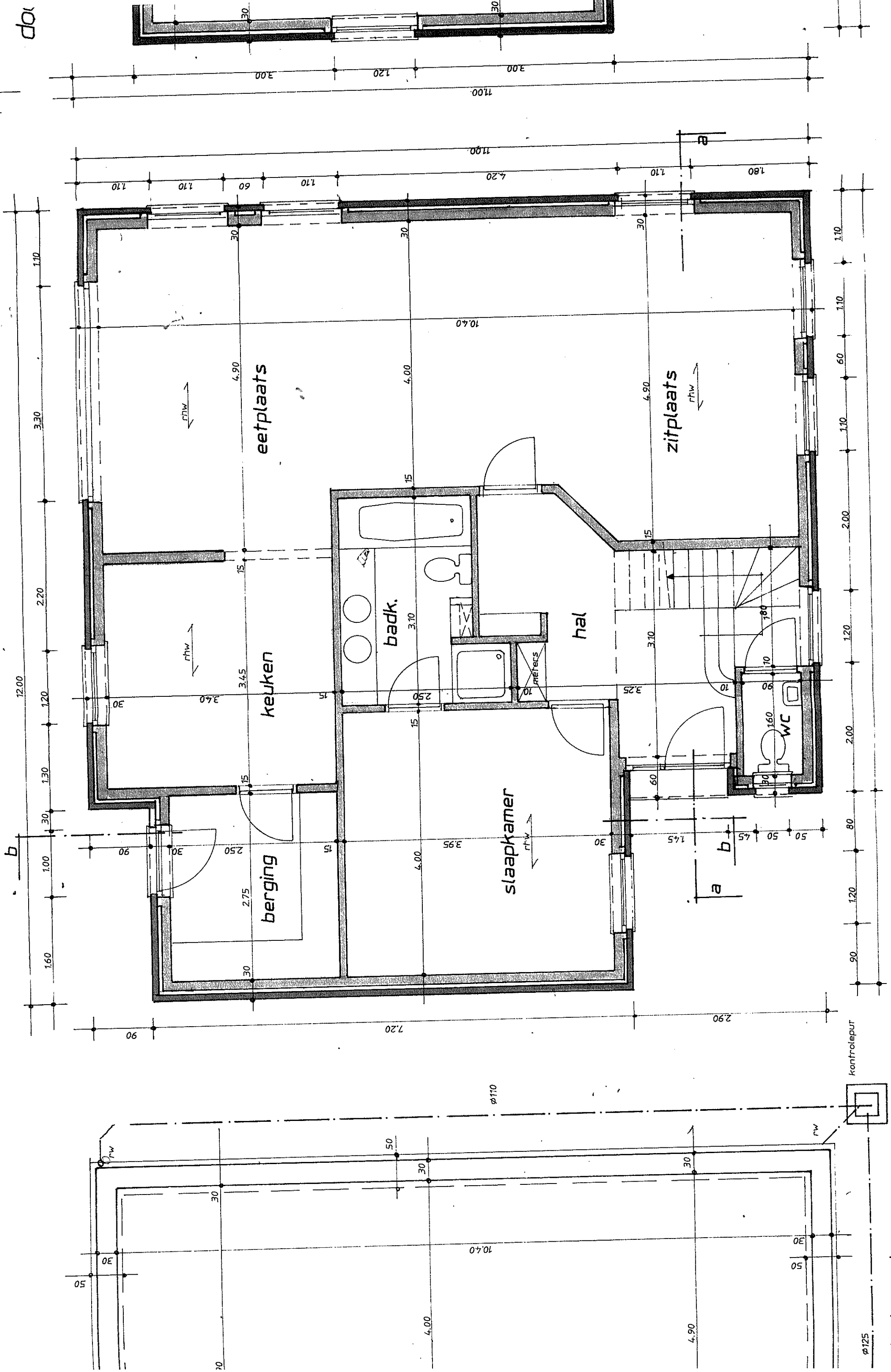
grondplan
