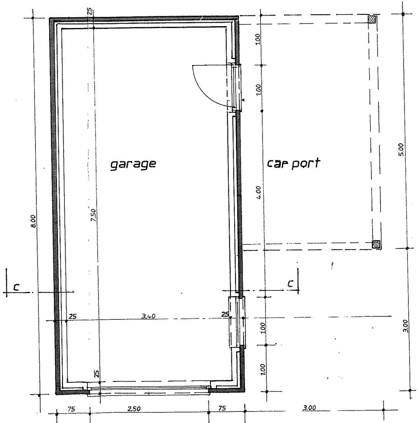
grondplan garage
