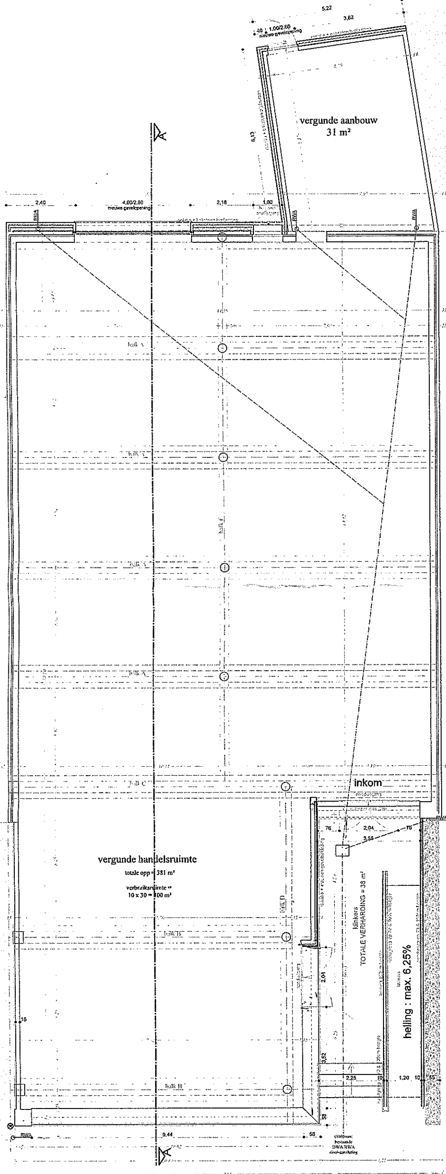
Plan Gelijkvloers.
