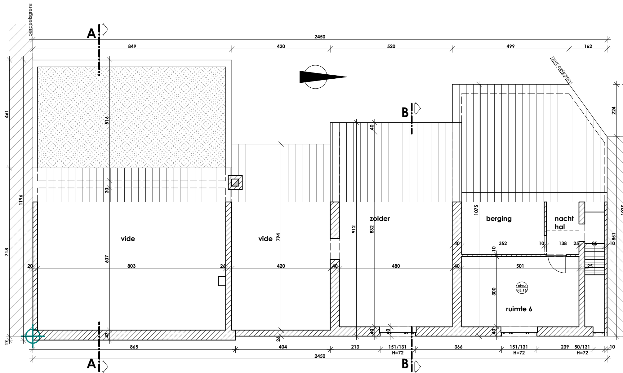
verdiepingsplan bestaande toestand
